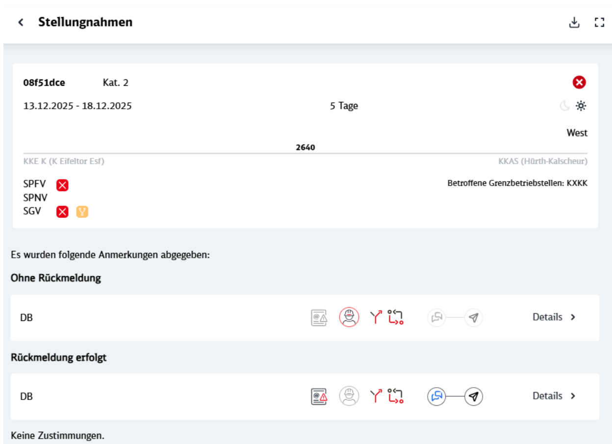
Abbildung 127: Stellungnahme-Liste
