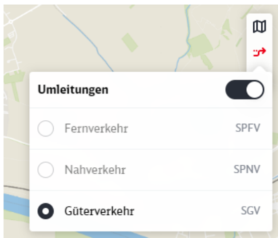
Abbildung 34: Umleitungen
