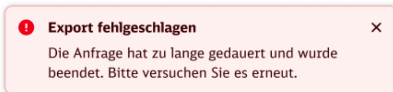
Abbildung 76: Fehlgeschlagener Export
