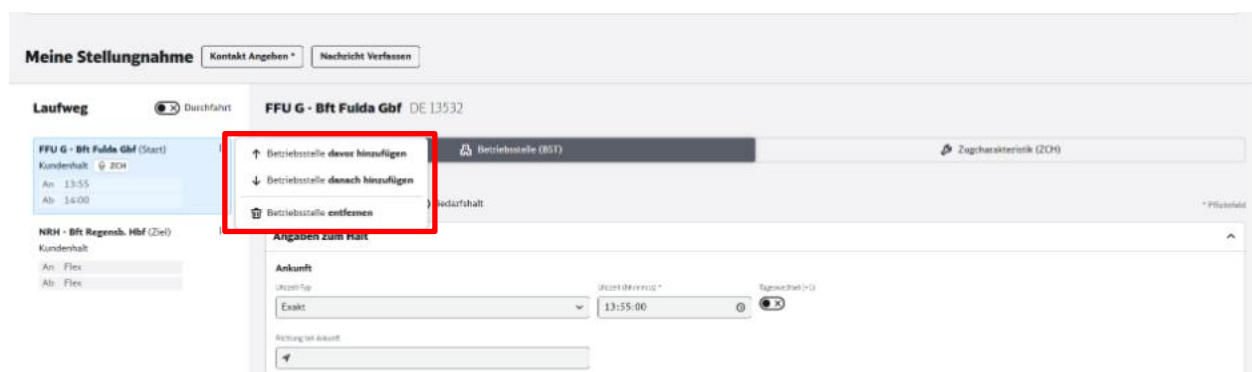
Abbildung 113: Laufweganpassung
