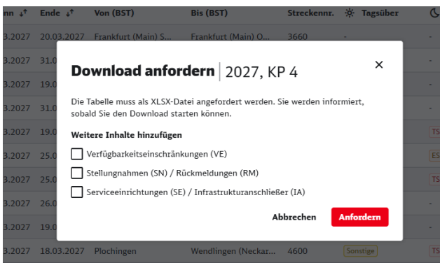
Abbildung 72: Exportmenü
