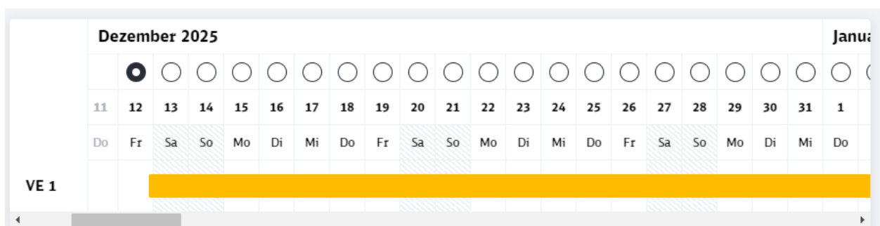
Abbildung 37: Kalender
