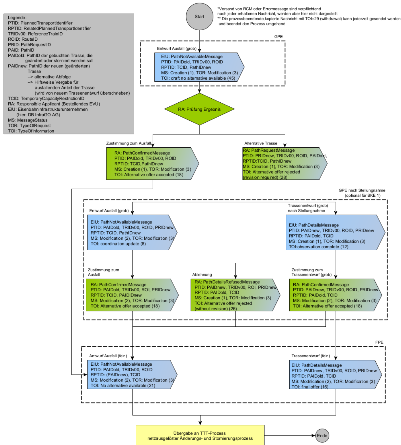
Abbildung 2: Nachrichtenabfolge Trassenausfall
