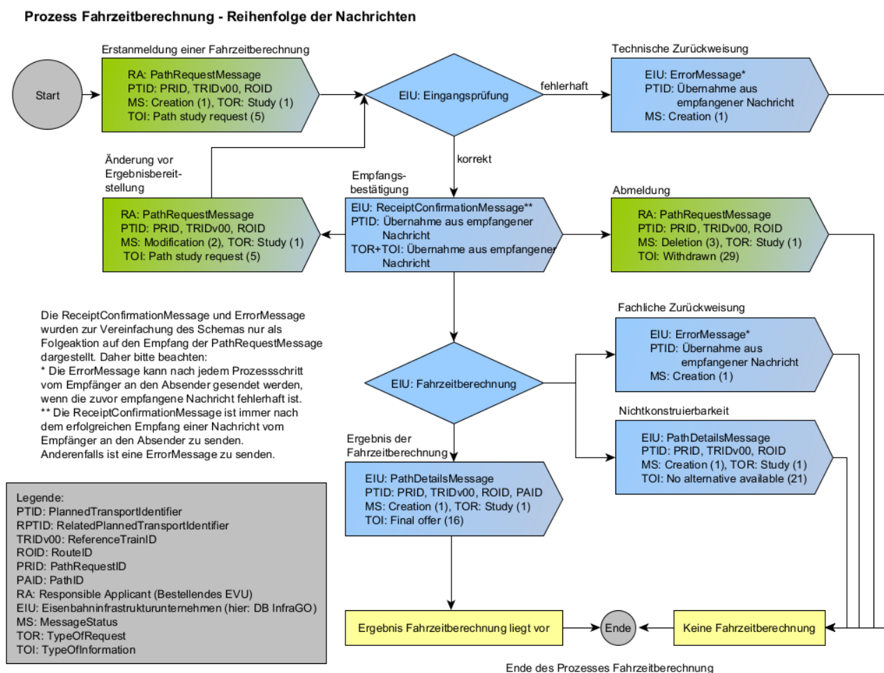
Abbildung 17: Geschäftsvorfallfolgen - Fahrzeitberechnungen
